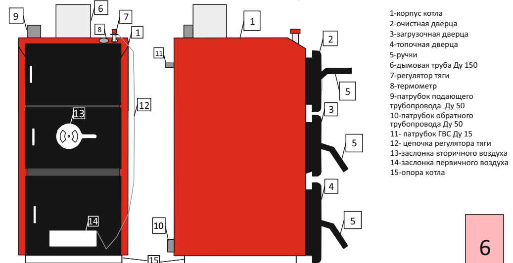
Рисунок 4. Основные элементы котлов DRAGON-TA
