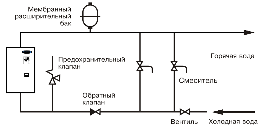
Рис.11 Упрощенная схема подключения в качестве котла с проточным режимом работы
