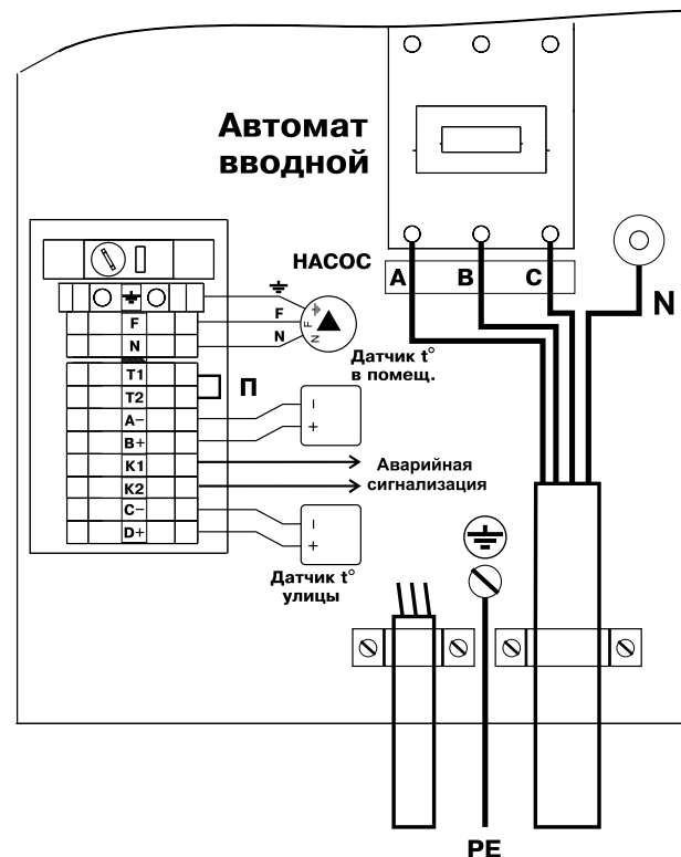
Рис.3 Схема подключения котла
