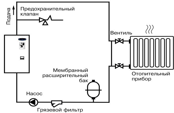
Рис.10 Упрощенная схема подключения котлом в отопительную систему с циркуляционным насосом
