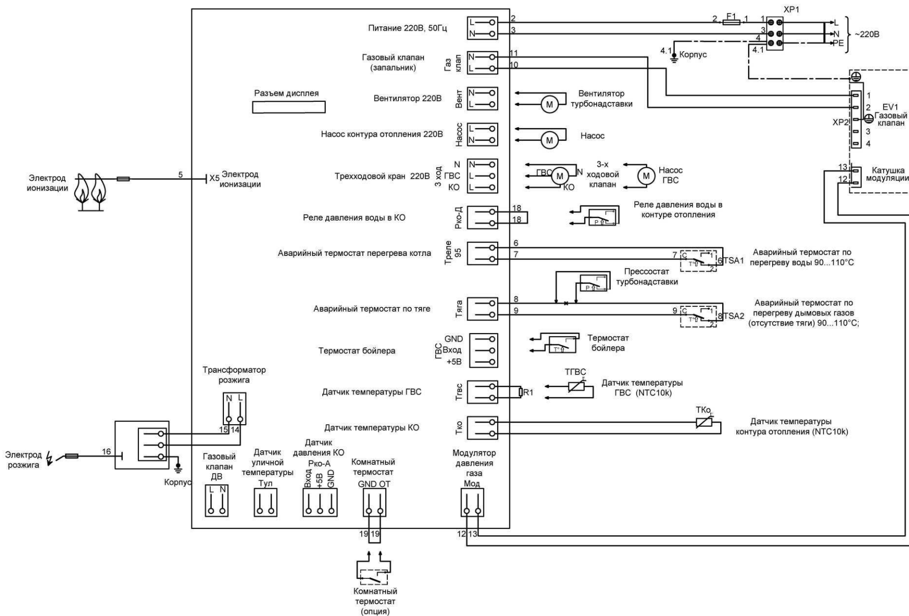
Рисунок 7. Электрическая схема котлов ТИТАН Z30М; Z40М; Z50М; Z60М, Z65М
