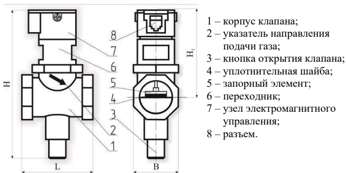
Рисунок 2 – Внешний вид клапанов КЗЭУГ
