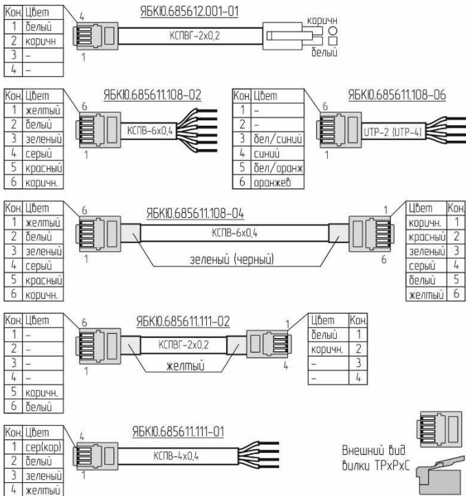
Рисунок Б.4 – Цветовая маркировка проводов кабелей
