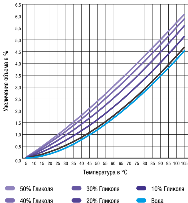
График №2 Температурное расширение системных жидкостей
