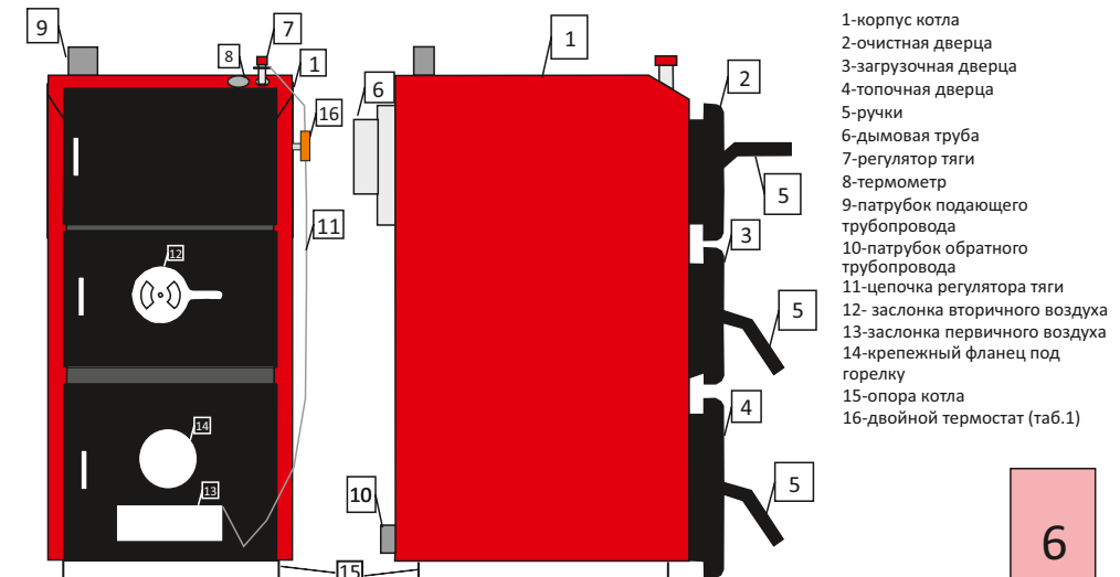
Рисунок 4. Основные элементы котлов DRAGON-KR
