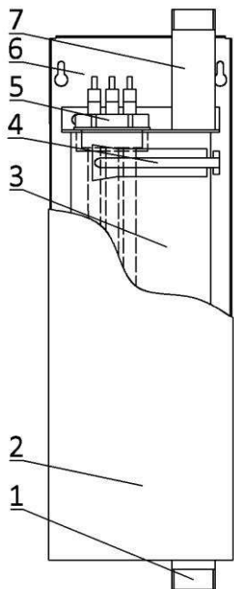
Рисунок 1. Схема электродкотла.
