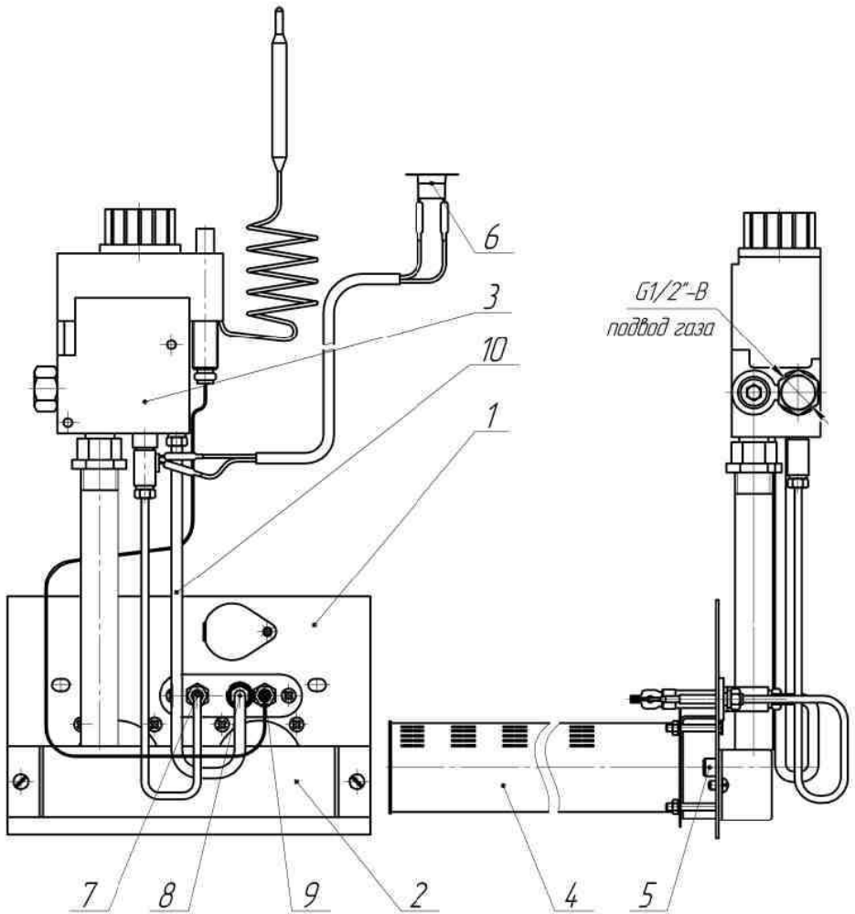
Рисунок 1 Устройство горелки котла
