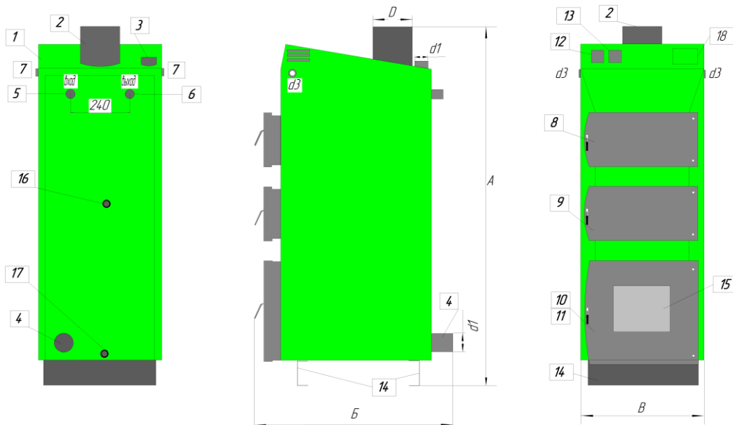
Рисунок 3. Основные размеры котлов Dragon BIO (SE/SLE)
