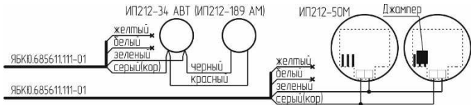
Рисунок Б.3 - схема электрическая подключения пожарных извещателей
