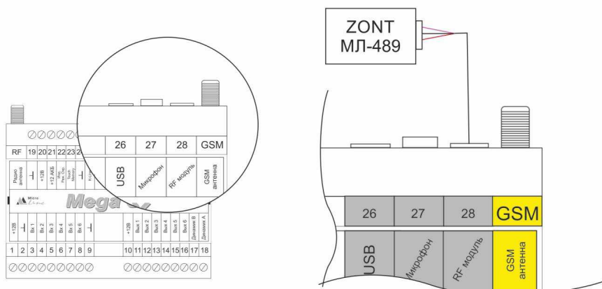
Подключение Радиомодуля МЛ-489
