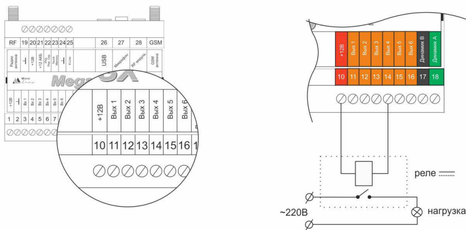
Подключение реле управления нагрузкой по выходу
