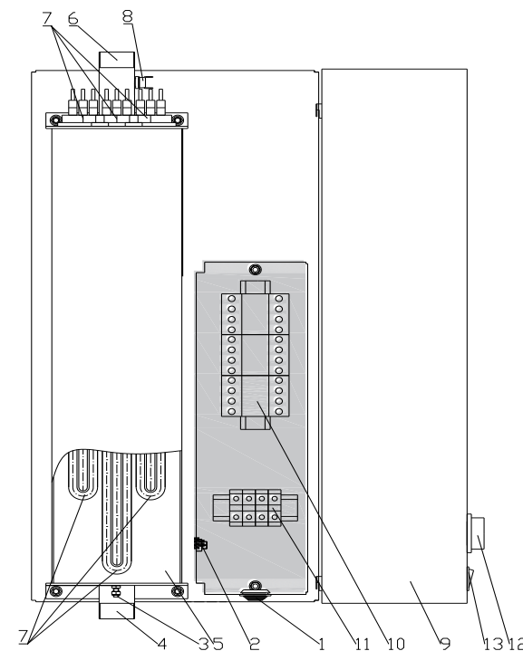
Рисунок 1. Устройство электродкотла. (крышка открыта)
