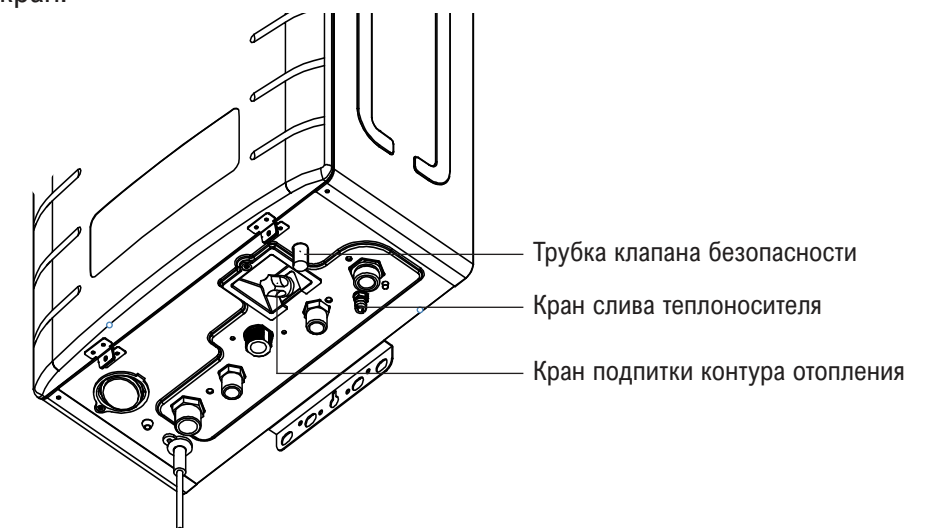
Рисунок 4. Схема нижней панели котла.
