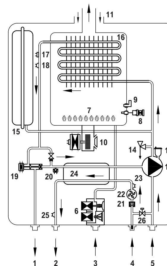
Рисунок 3. Функциональная схема котла.
