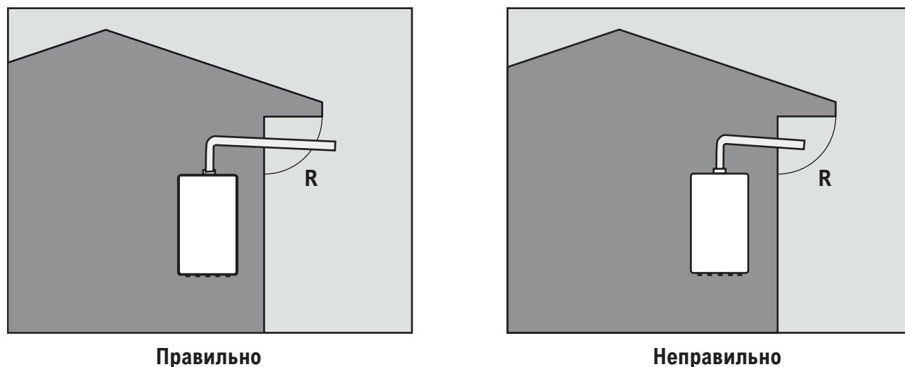
Рисунок 8. Зона повышенного давления воздуха.
