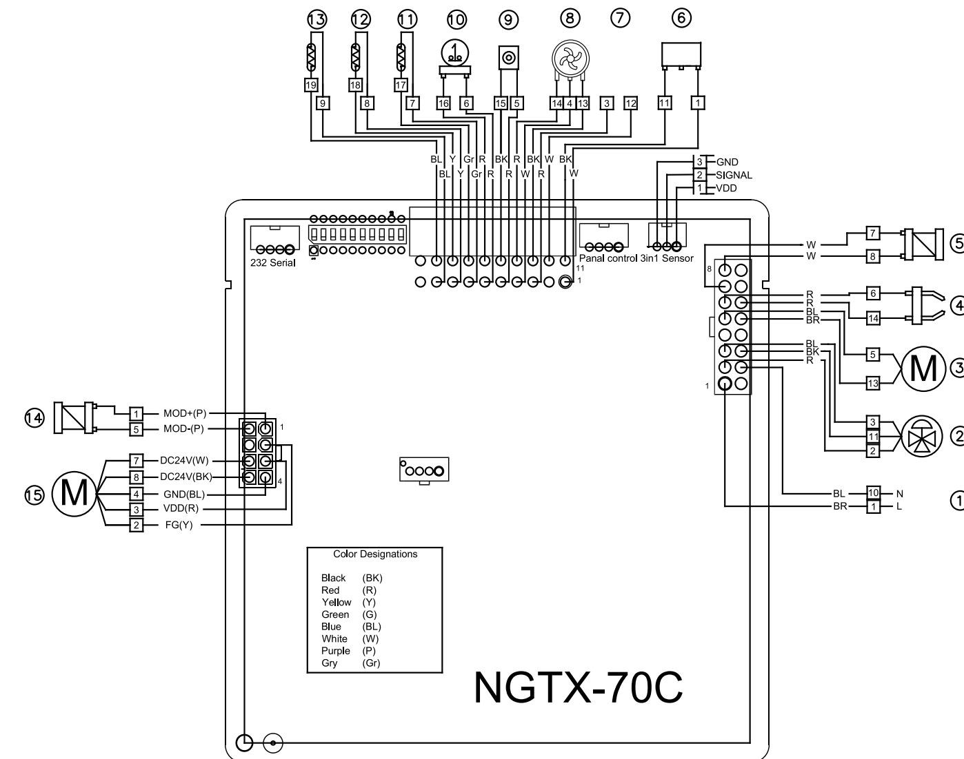
Рисунок 13. Схема электрическая.
