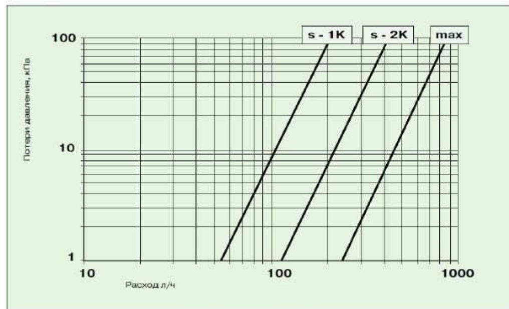
Диаграмма 2 Прямой
