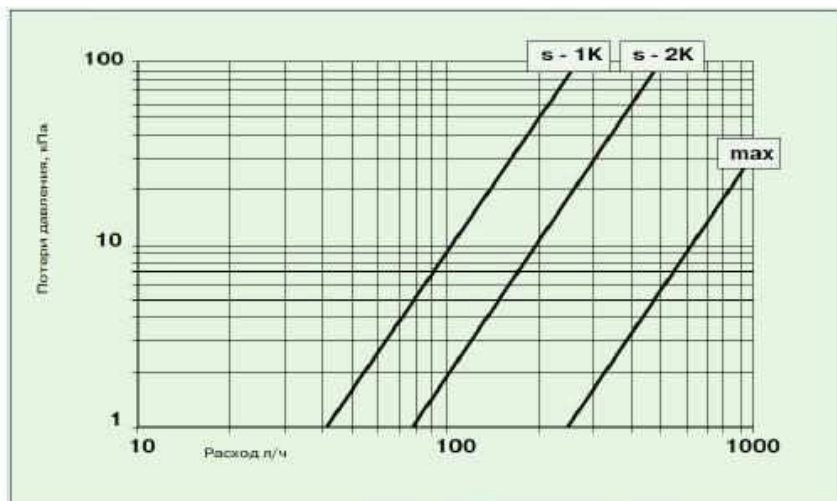
Диаграмма 1 (Угловой)
