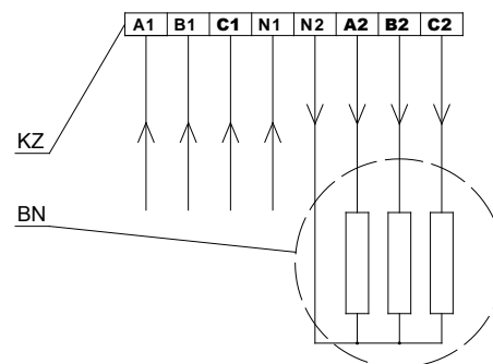
Рис.1а. Пример трехфазного подключения ТЭНБ-6, ТЭНБ-9
