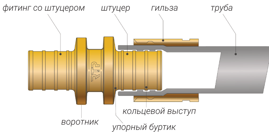
Рис. 4. Конструкция аксиальных фитингов
