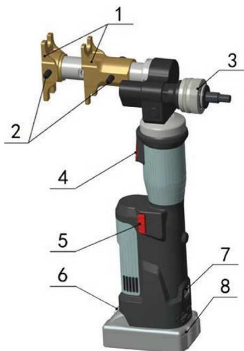
Рис. 2. Внешний вид в сборе
