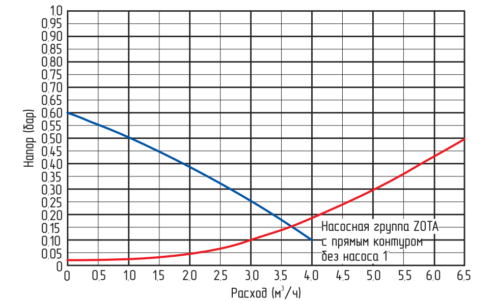
Рис.1 Гидравлические характеристики.
