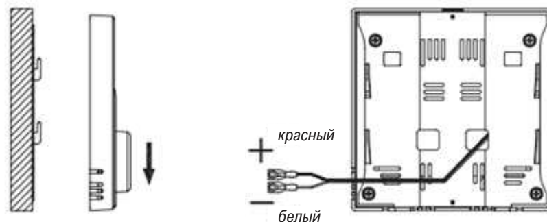
Рисунок 15. Подключение пульта управления NCTR-60R.
