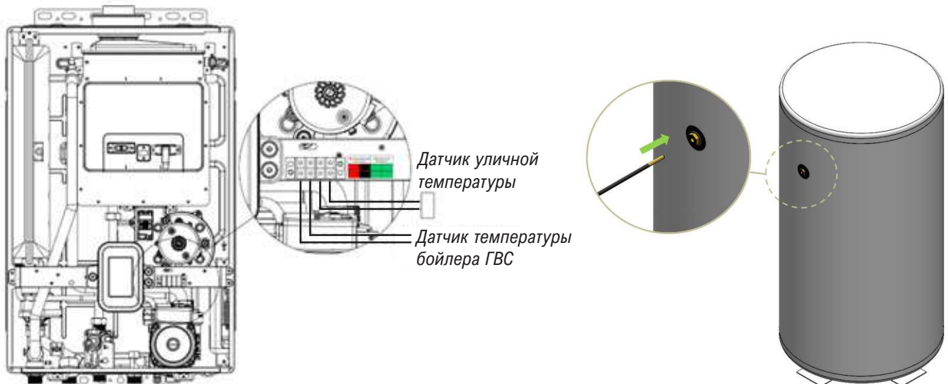
Рисунок 14. Подключение датчика температуры ГВС в бойлере.
