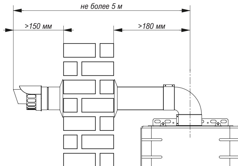
Рисунок 12. Коаксиальный дымоход.
