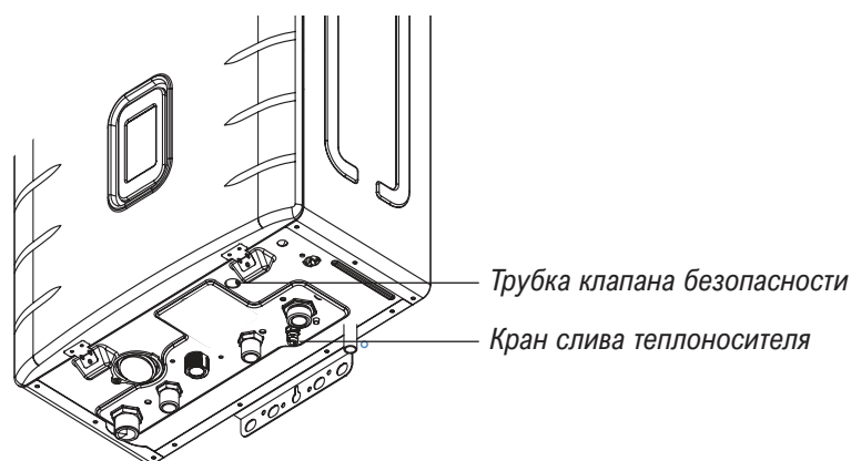
Рисунок 4. Схема нижней панели котла.
