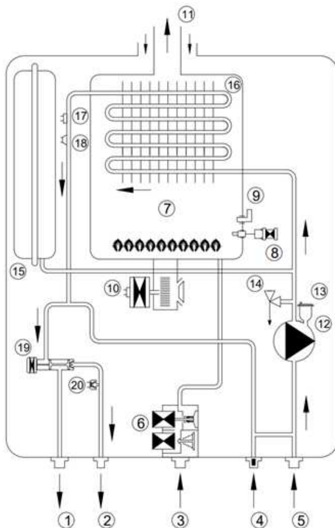
Рисунок 3. Функциональная схема котла.
