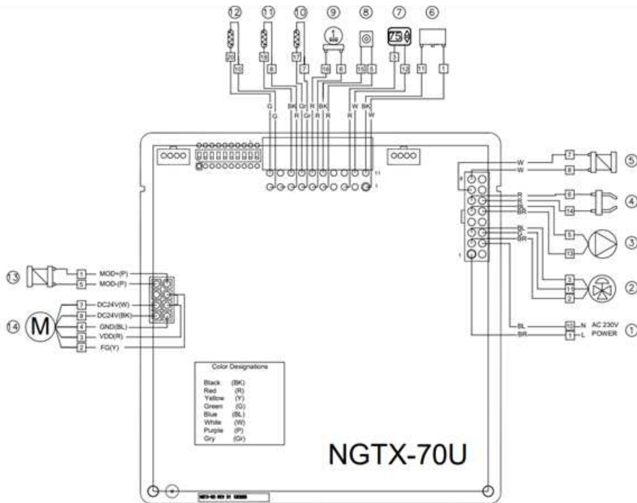
Рисунок 16. Схема электрическая.
