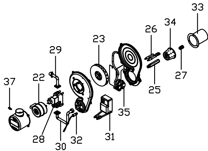
Горелка TGB-18/20
