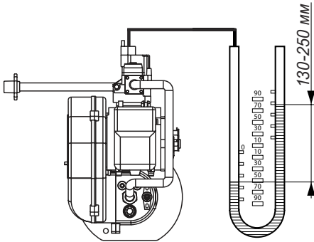
Рисунок 13. Проверка номинального давления подачи природного газа.
