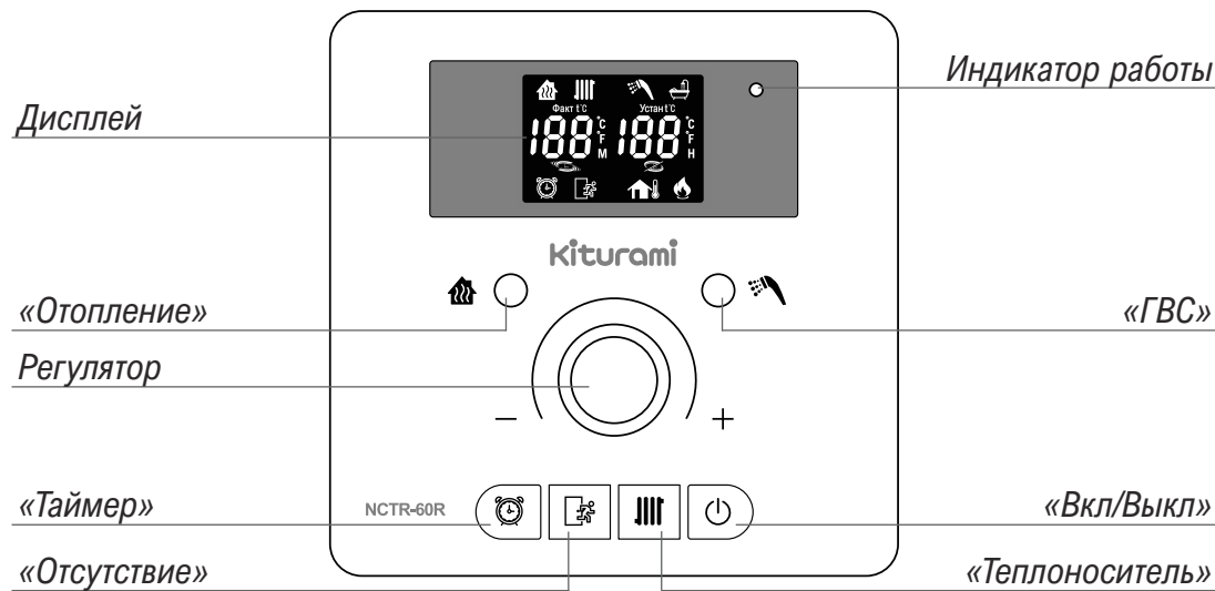
Рисунок 5. Дисплей и кнопки управления NCTR-60R.
