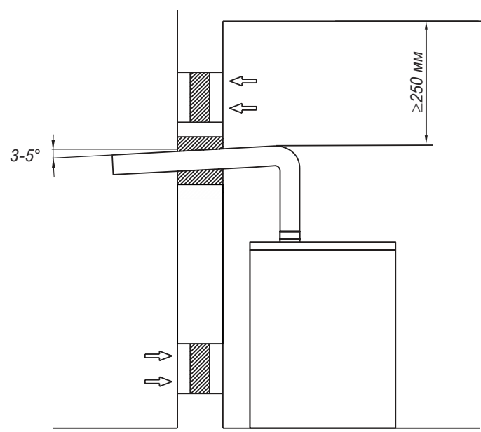
Рисунок 8. Система дымоудаления.
