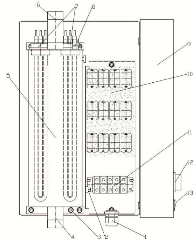
Рисунок 1. Устройство электродкотла. (крышка открыта)
