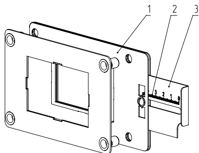
Рис.14 Заслонка вентилятора
