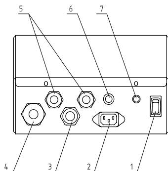
Рис.8 Расположение органов управления на задней панели пульта
