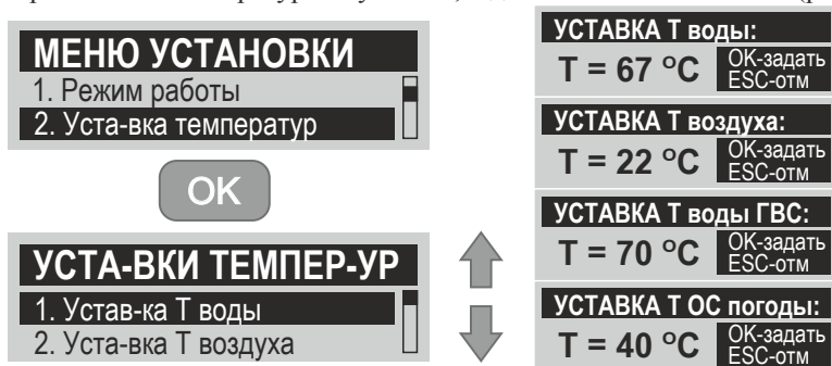
Рисунок 18 Установка температурных параметров
