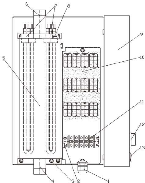
Рисунок 1. Устройство электрокотла (крышка открыта)
