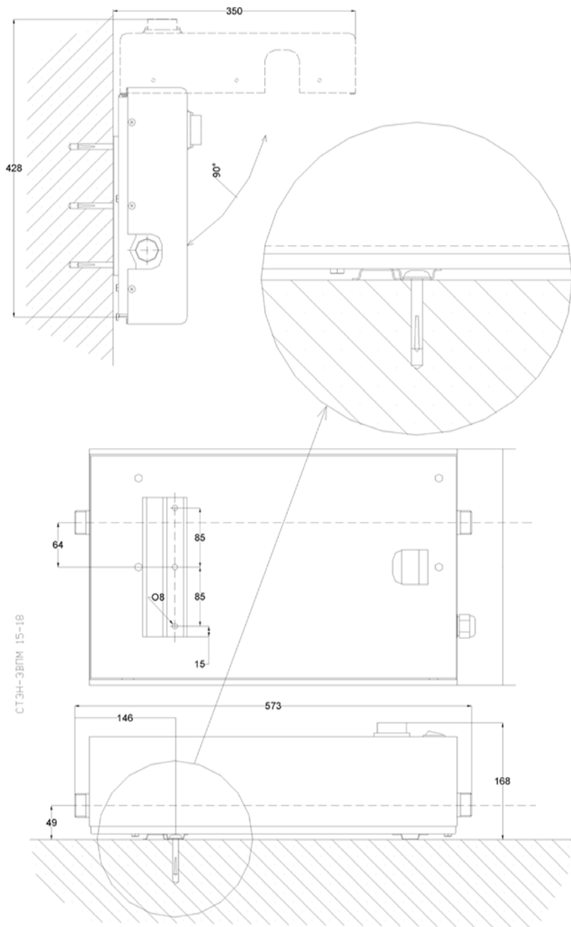
Рисунок 3. Установочные размеры
