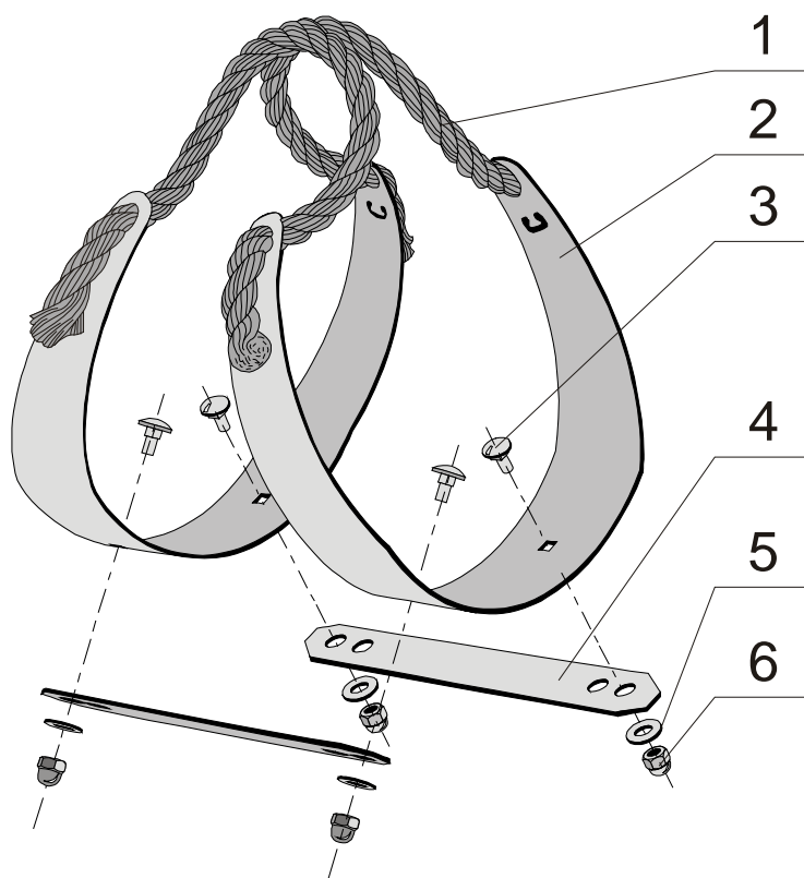
Рисунок 1. Сборка дровницы
