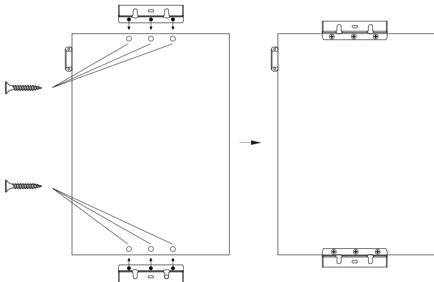
Рис.10 Монтаж кронштейнов ZOTA Joy 36 кВт
