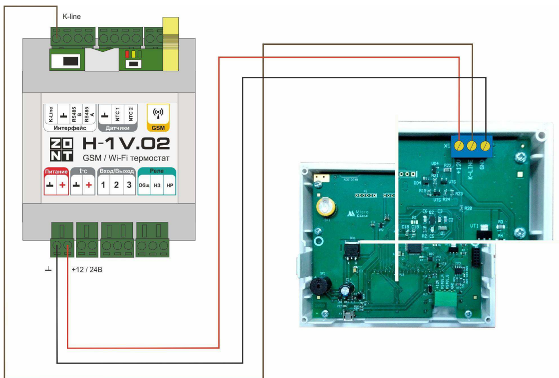
Интерфейс K-Line
