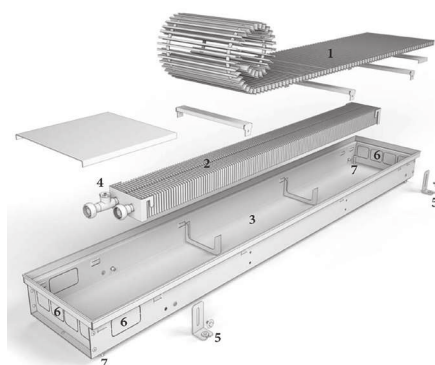
Рис. 1. Устройство внутрипольного вентилляторного конвектора типа SCN
