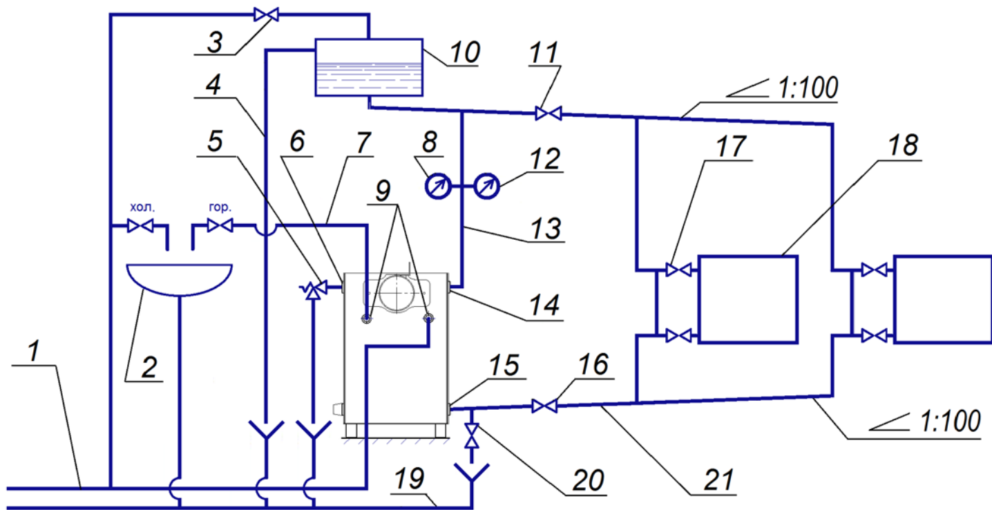
Рисунок 8. Схема монтажа котла в однотрубной системе отопления с верхней разводкой, естественной циркуляцией, открытым расширительным баком, для одноэтажных строений:
