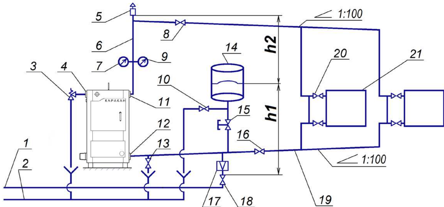
Рисунок 9. Схема монтажа котла в однотрубной системе отопления с верхней разводкой, естественной циркуляцией, мембранным расширительным баком, для одноэтажных строений:
