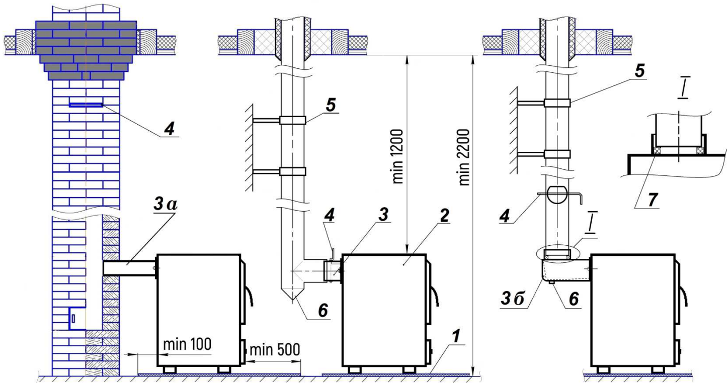
Рисунок 5. Монтаж котлов, имеющих выход дымохода «назад»:
