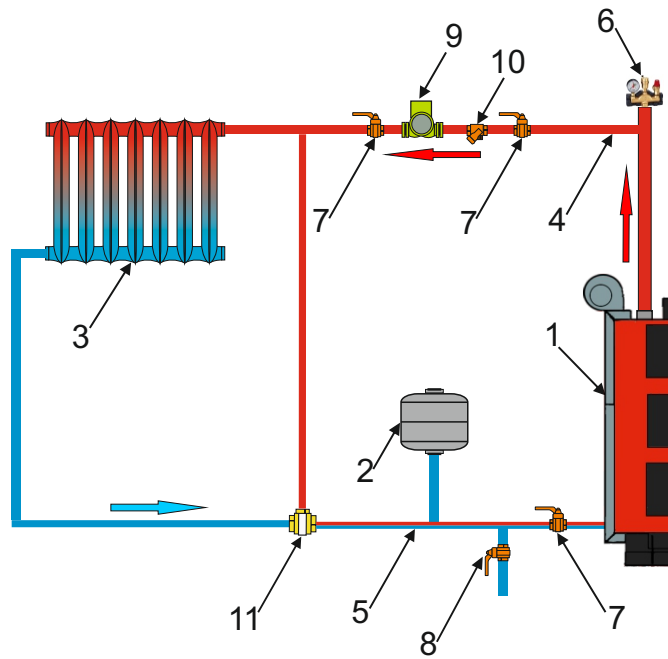
Рисунок 2.1. Схема присоединения котла к системе отопления закрытого типа: 1-котел 2-расширительный бак (закрытого типа) 3-радиатор системы отопления 4-подающий трубопровод 5-обратный трубопровод 6-группа безопасности котла 7-кран системы отопления 8-кран слива воды 9-циркуляционный насос 10-фильтр-отстойник 11-термостатический смесительный клапан
