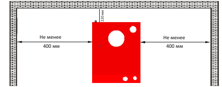
Рисунок 5. Установка котла в помещении котельной.
