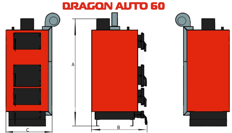
Рисунок 3. Основные размеры котлов DRAGON-Auto
