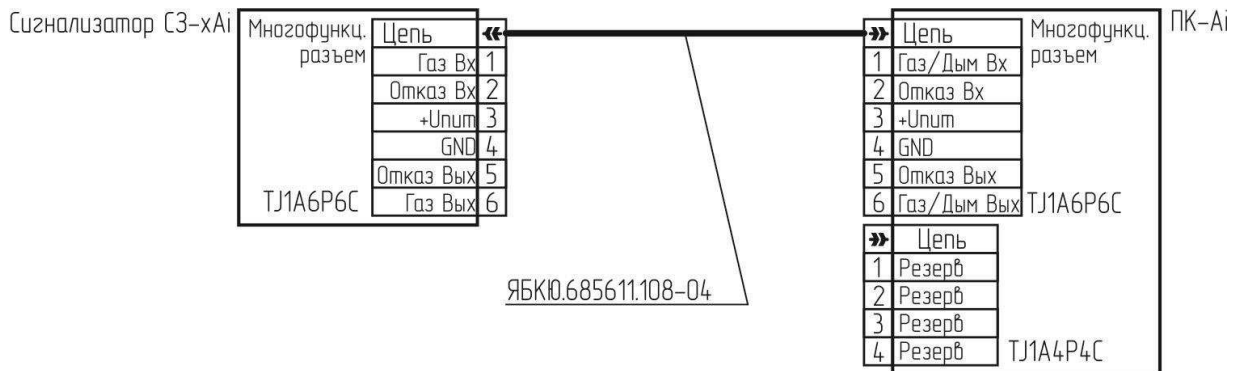
Рисунок 1 – Типовая схема подключения
